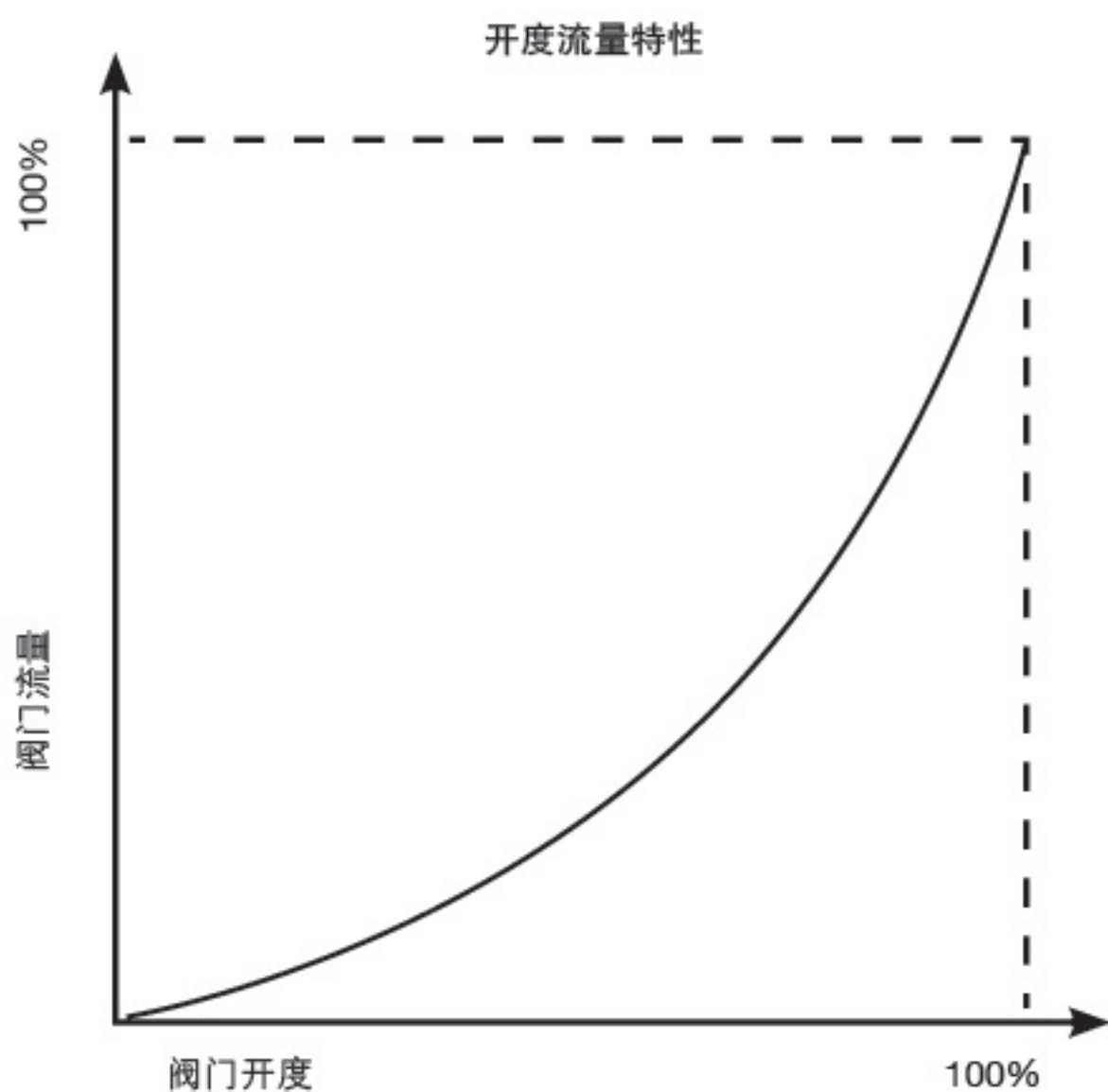
等百分比流量特性
